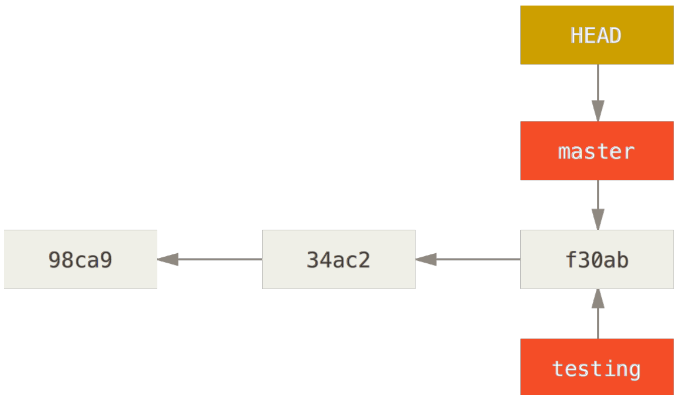
Figure 13. HEAD pointant vers une branche
