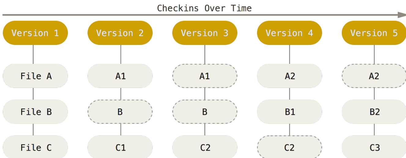
Figure 5. Git stocke les données comme des instantanés du projet au cours du temps.
