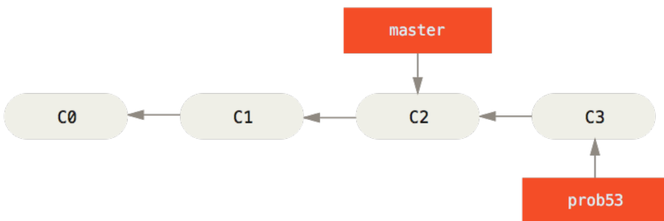
Figure 20. La branche prob53 a avancé avec votre travail
