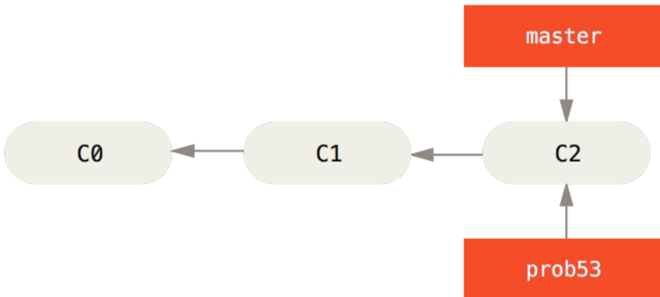
Figure 19. Création d'un nouveau pointeur de branche
