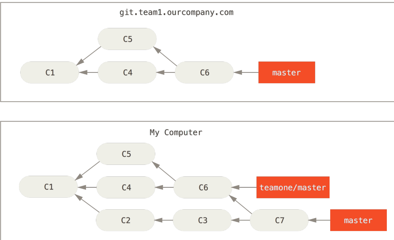
Figure 45. Récupération de commits et fusion dans votre copie
