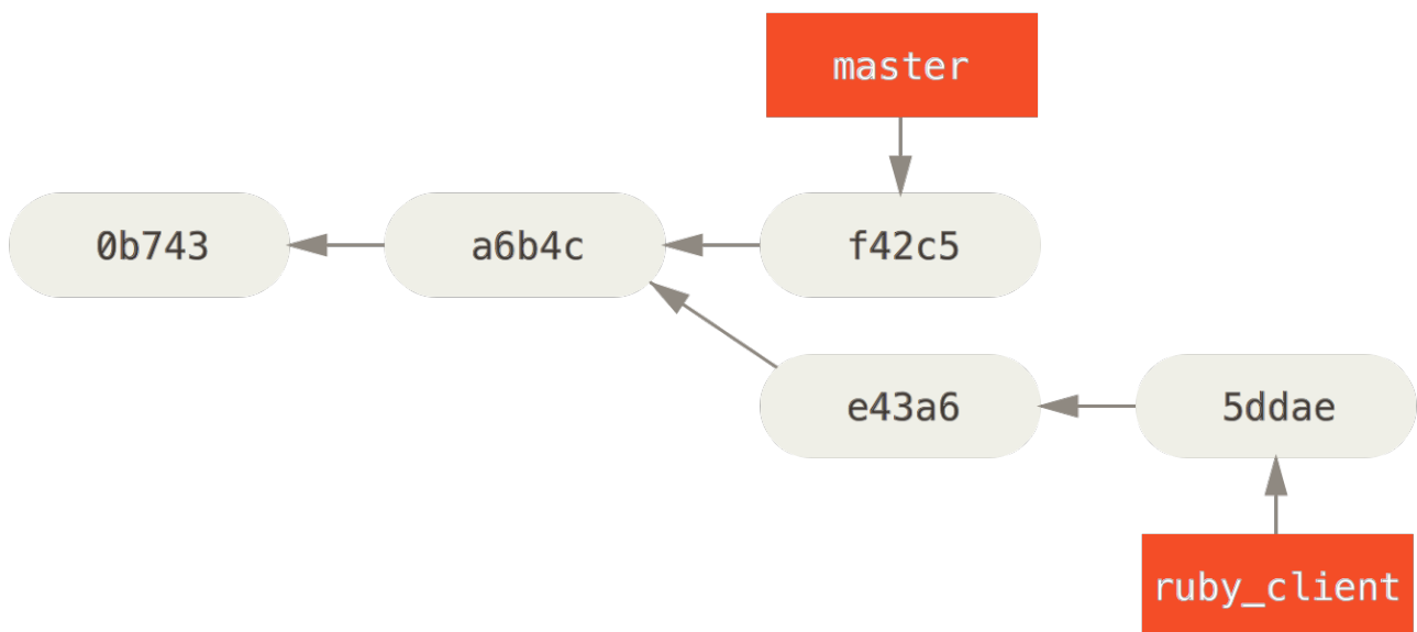
Figure 80. Historique d'exemple avant une sélection.
