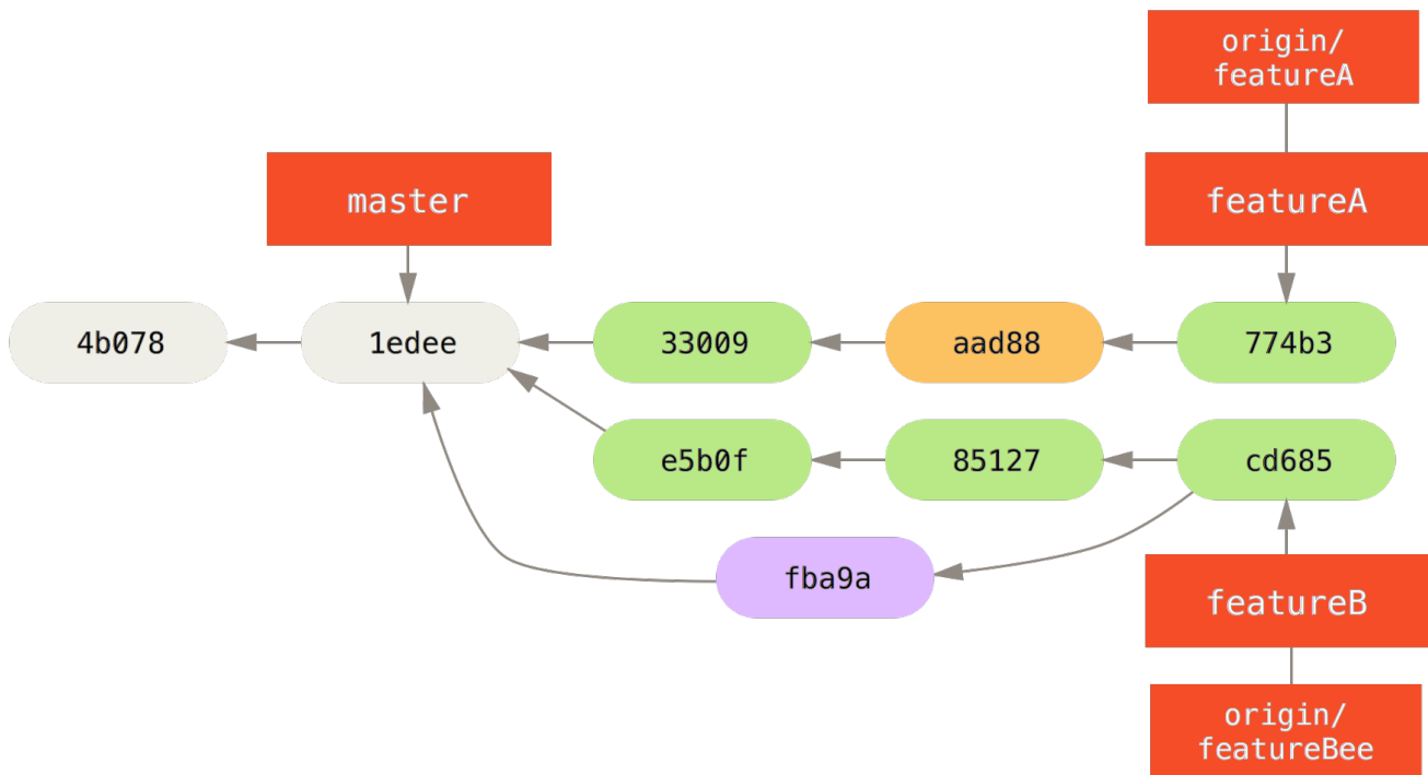
Figure 67. L'historique de Jessica après la validation dans la branche thématique.
