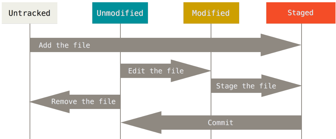
Figure 8. Le cycle de vie des états des fichiers.
