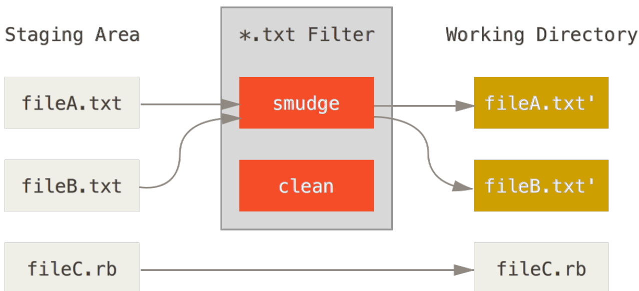
Figure 144. Le filtre « smudge » est lancé lors d'une extraction.
